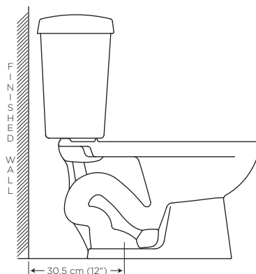
Distance between wall and the hole / Distancia entre la pared y el agujero del desagüe
